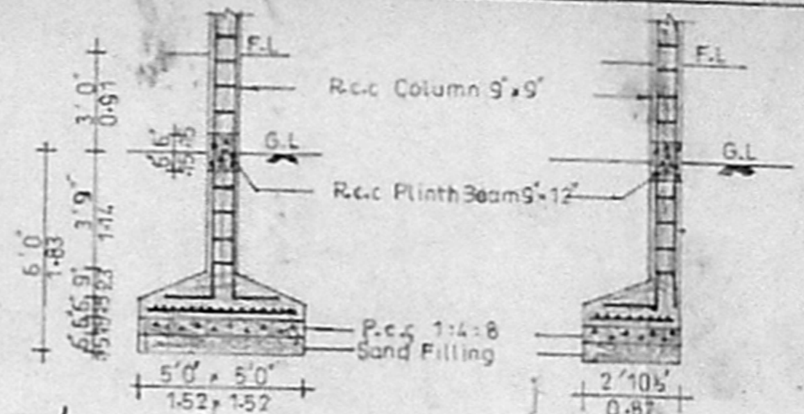
C.S. OF COLUMN scale: 1:50
