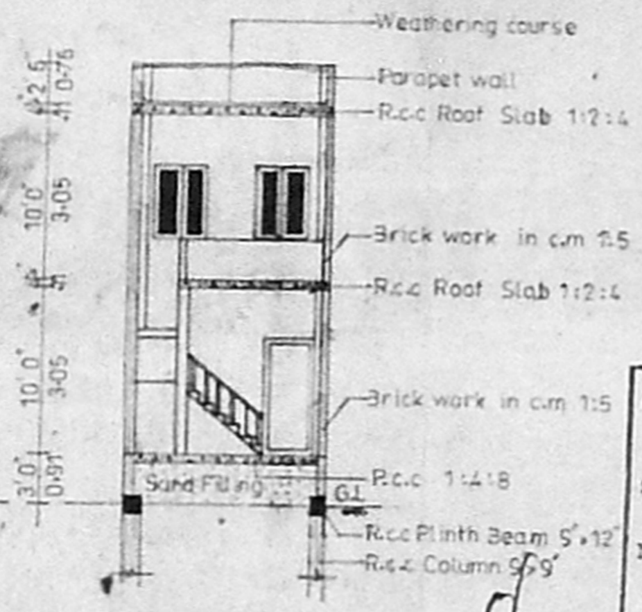
SECTION ON A3
